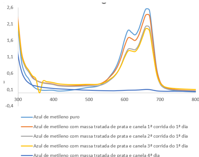
Figura 02 - Espectros no UV-vis do acompanhamento da degradação do corante azul de metileno na presença do composto do sal de prata tratado por biossíntese.
