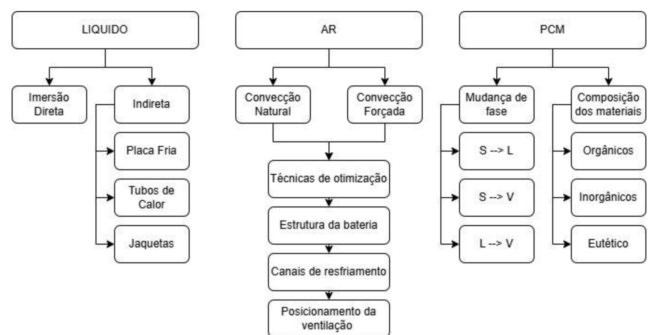
Fig.1- Classificação BTMS dependendo do meio de resfriamento
